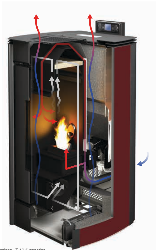
sezione .IT 10,5 ermetica
